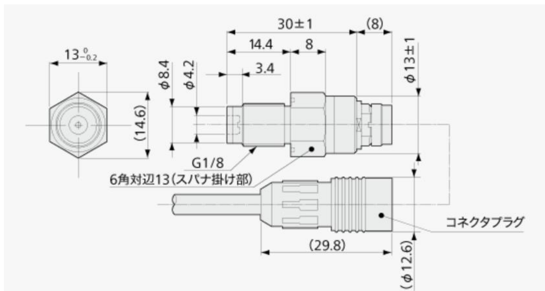
外形尺寸图
