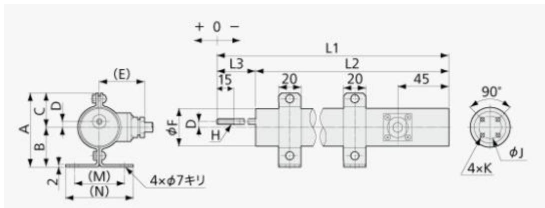
外形尺寸图
