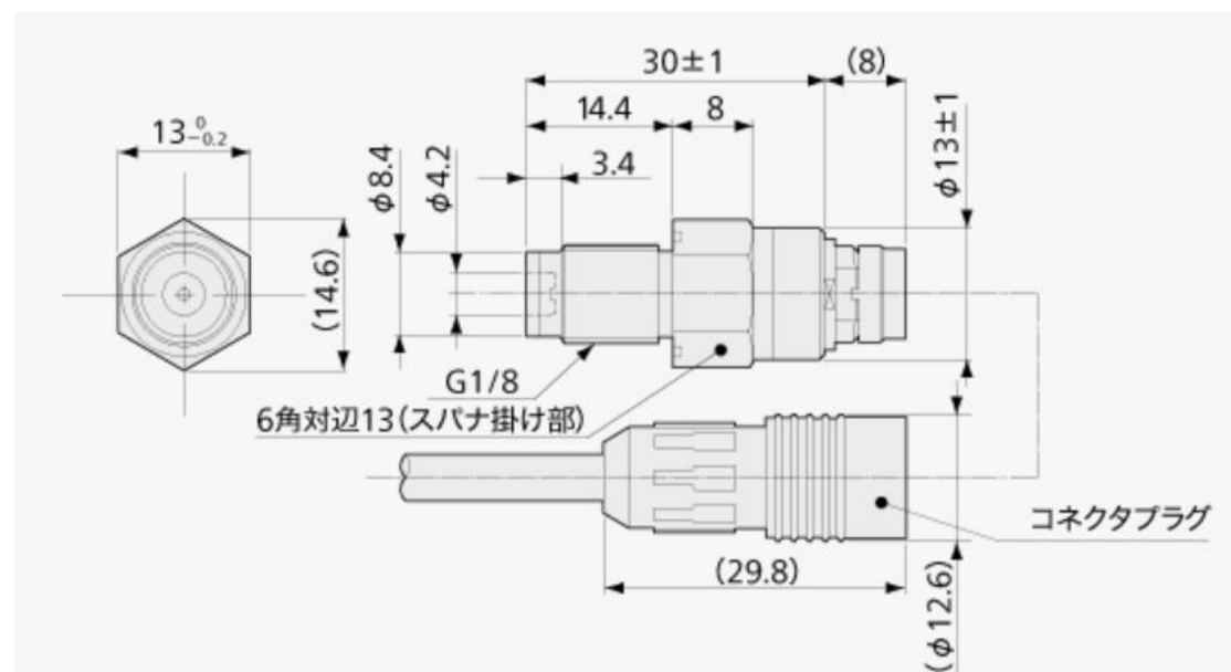
外形尺寸图
