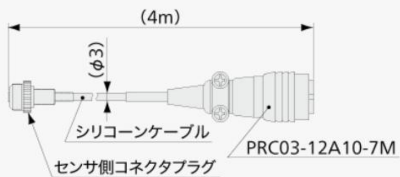
標準ケーブル(別売品)
