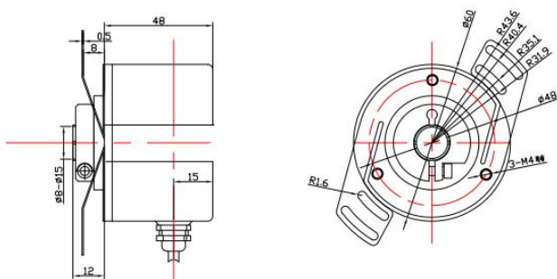
60mm 外径 8-15mm 孔径可选 20mm 孔深 轴向出线可选
