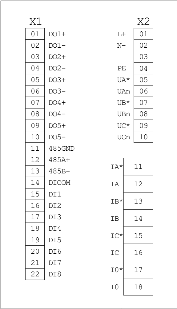
图 5.1 AM2SE-V 电气接线图（-H 和-V 背后端子定义完全相同）
