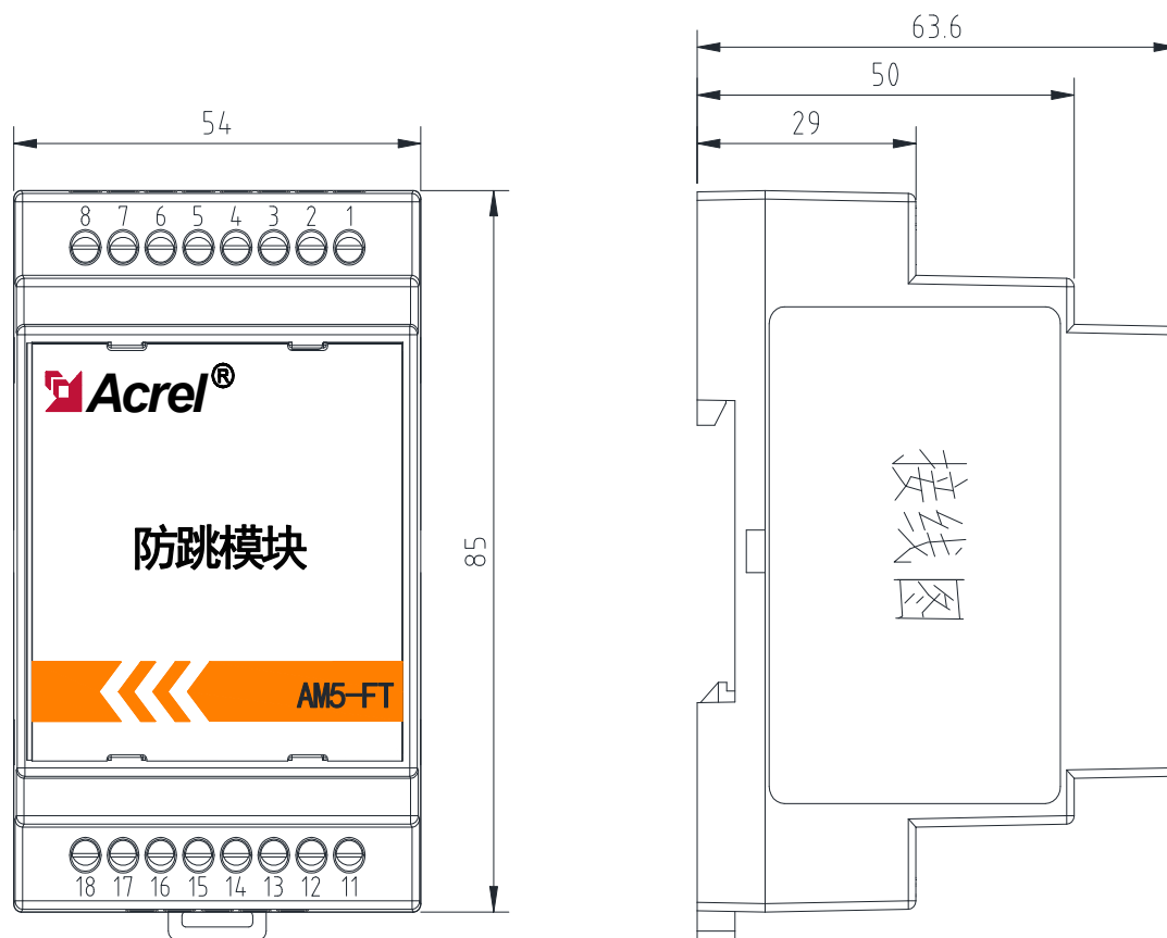
图 3 AM5-FT 尺寸图
