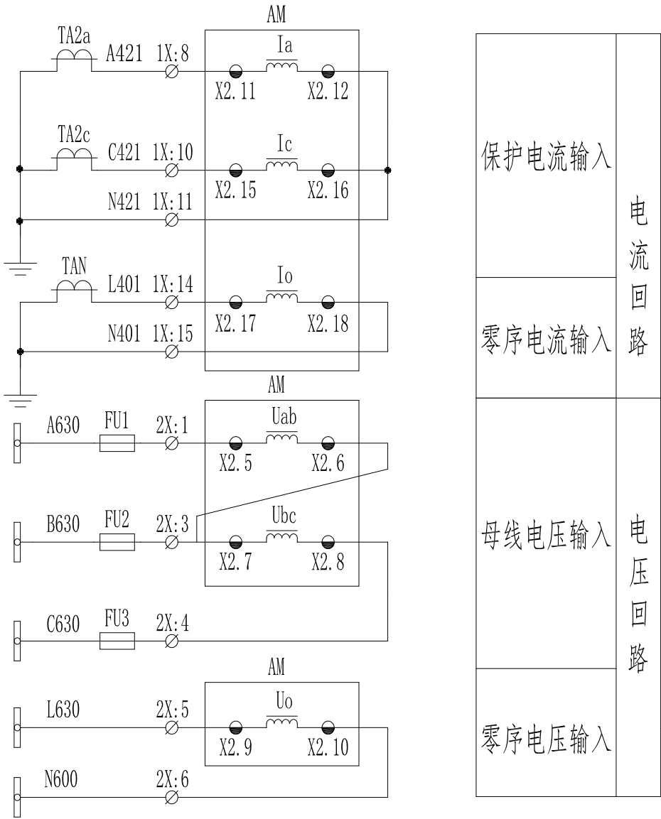
图 5.2 2PT 2CT 接线方法
