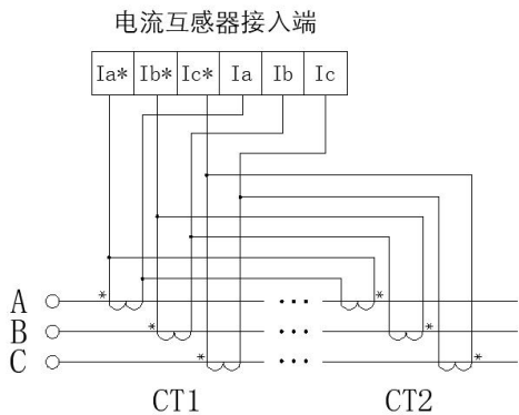
图8 两组互感器接法
