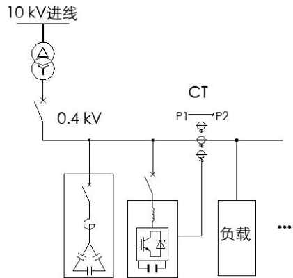
图4 一组互感器CT接法
