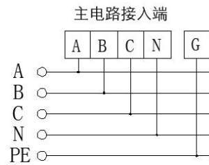
图7 主电路接法
