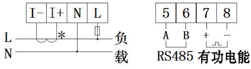
20 (100) A 规格接线图
