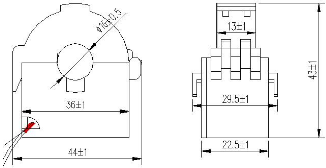
外置互感器外形尺寸
