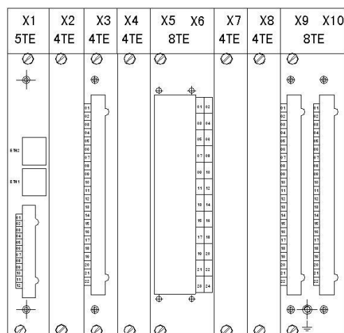
ARB5-M(ARB5-E)后面板示意图
