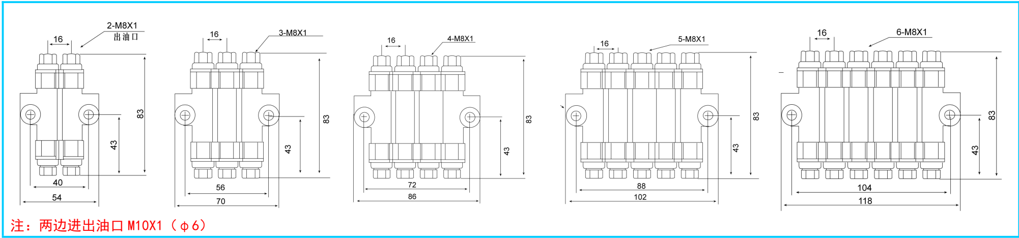
TH 型检知容积式分配器外形图
