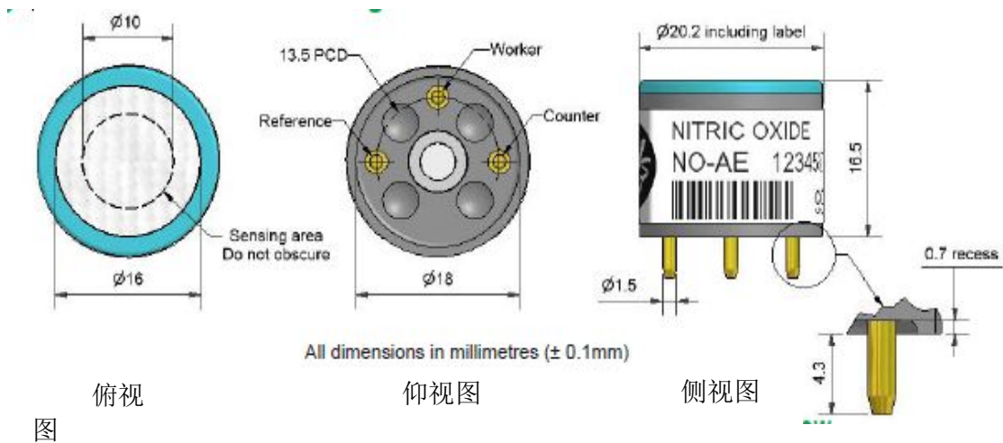
图1 NO-AE示意图
