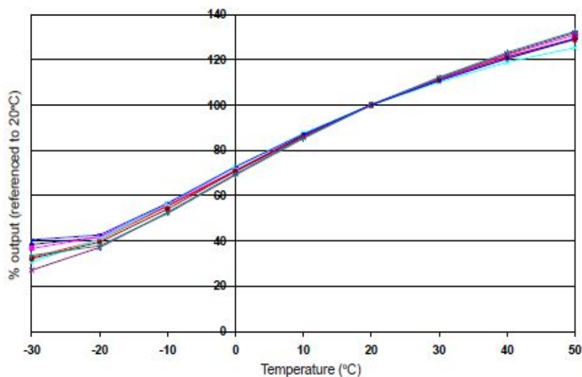
图1 CO通道灵敏度温度特性
