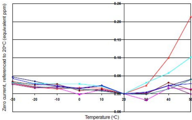
图7 H 2 S通道零点温度特性
