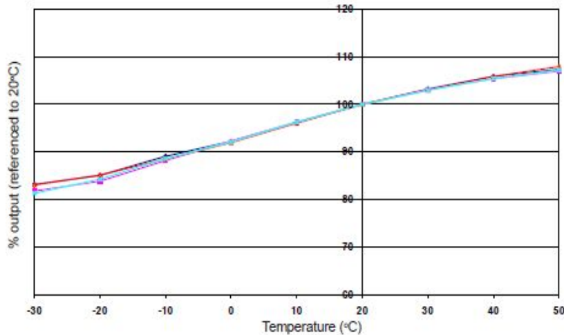
图6 H 2 S通道灵敏度温度特性
