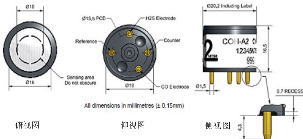
图4 传感器图示
