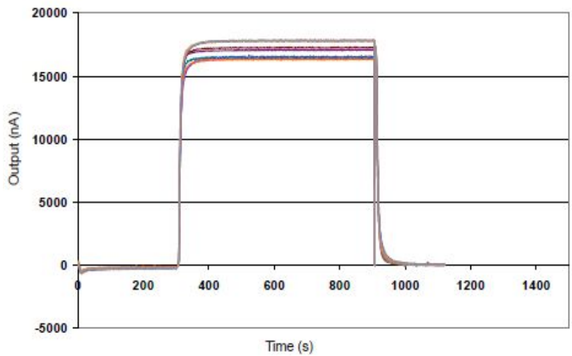
图5 H 2 S通道对25ppmH 2 S的反应
