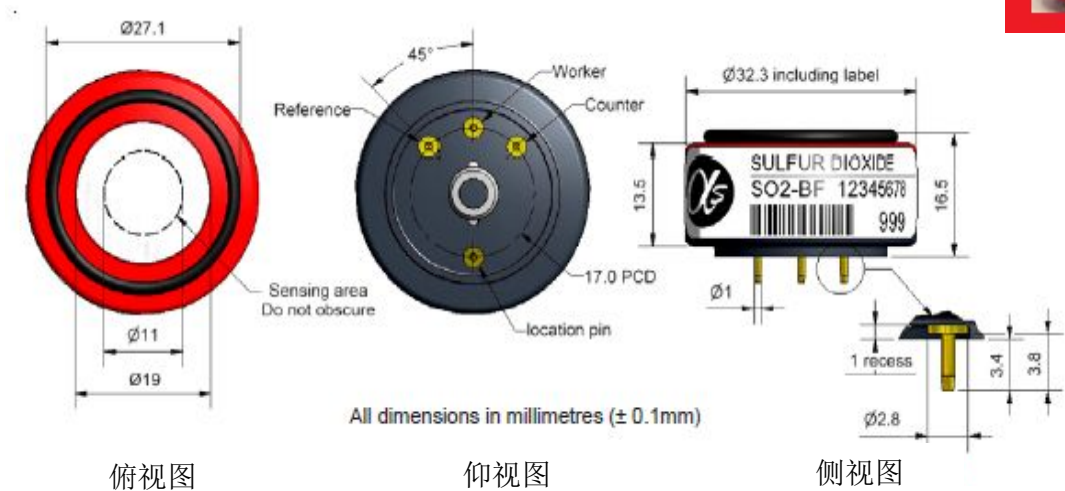
图1 SO2-BF示意图
