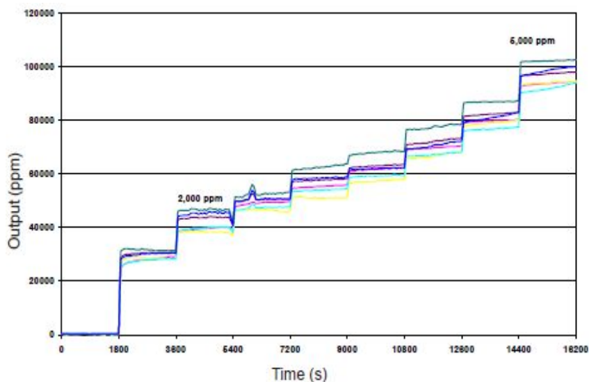
图4 过载线性度
