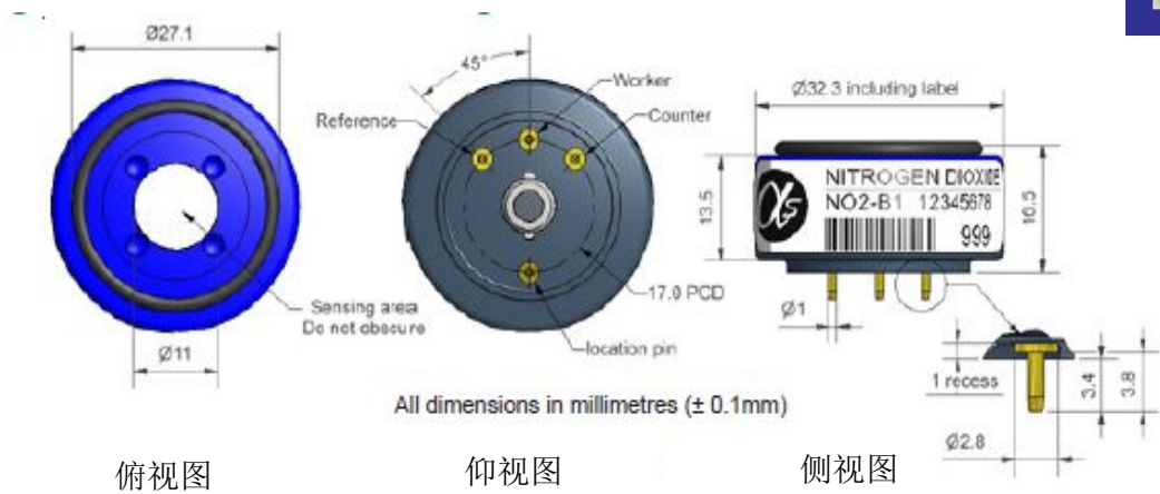
图1 NO2-B1示意图
