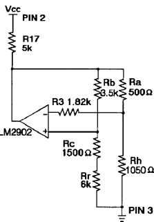
图 3 差分放大电路
