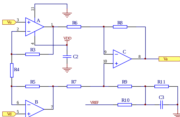
图三，差分放大电路
