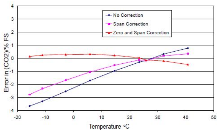
图4 温度补偿
