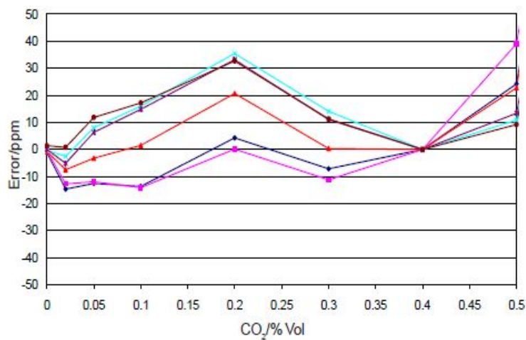
图5 线性度
