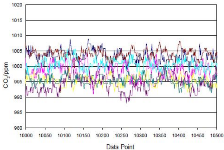
图6 分辨率
