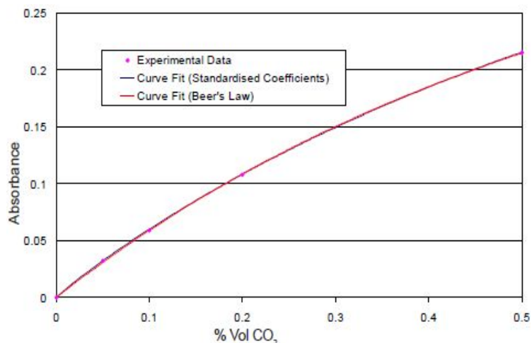
图3 比尔-朗伯特特性
