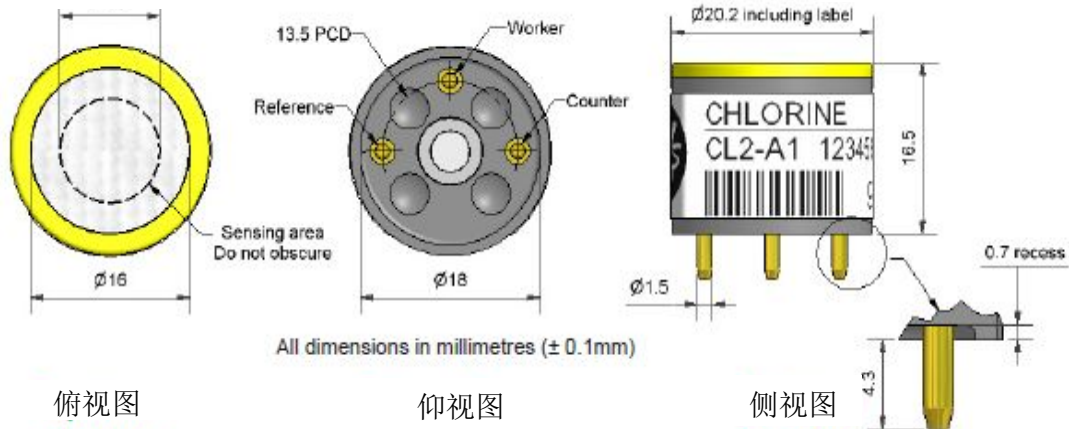
图1 CL2-A1示意图
