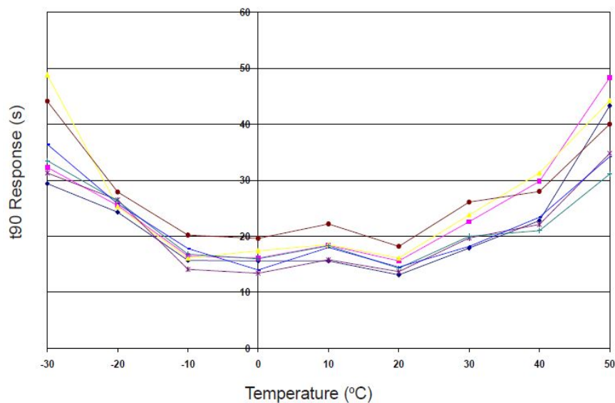
图4 对10ppm氯气的反应，受温度影响
