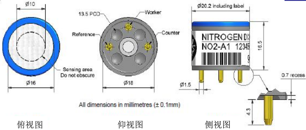
图1 NO2-A1示意图
