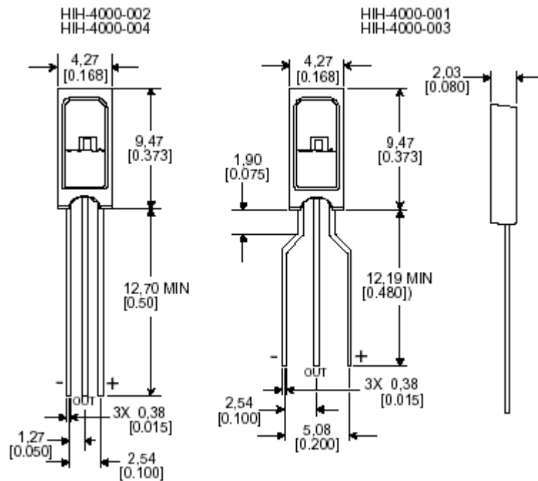
图 5: 安装尺寸 仅供参考 单位 mm (in)
