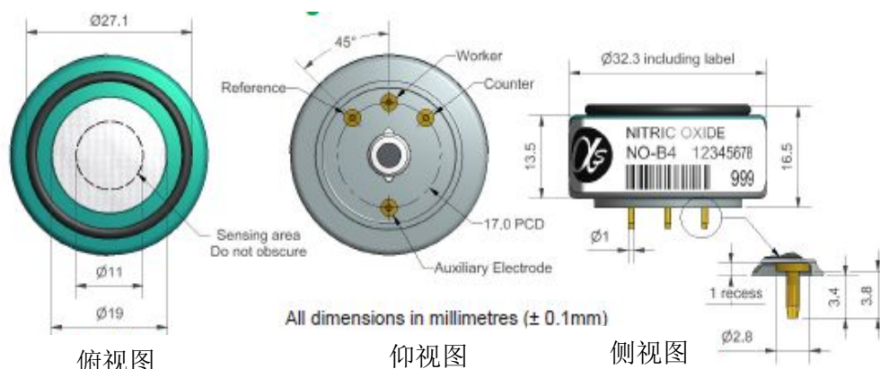
图1 NO-B4示意图
