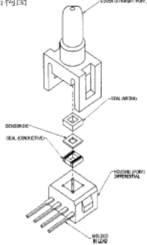
内部结构图
