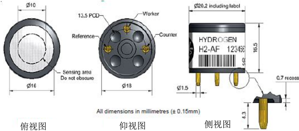
图1 H2-AF示意图
