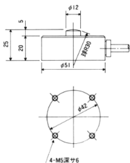
寸 法 図
