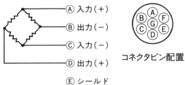
コネクタ接続図
