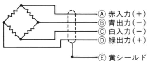
4芯ケーブル接続図
