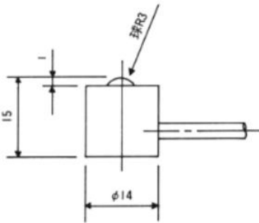
寸 法 図
