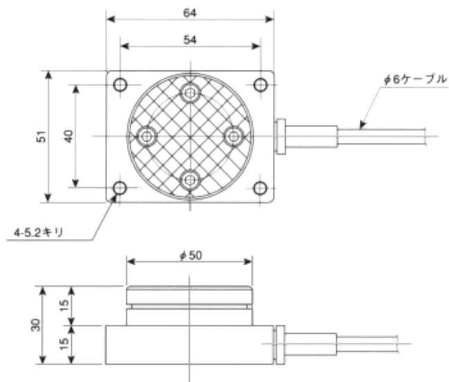
寸 法 図
