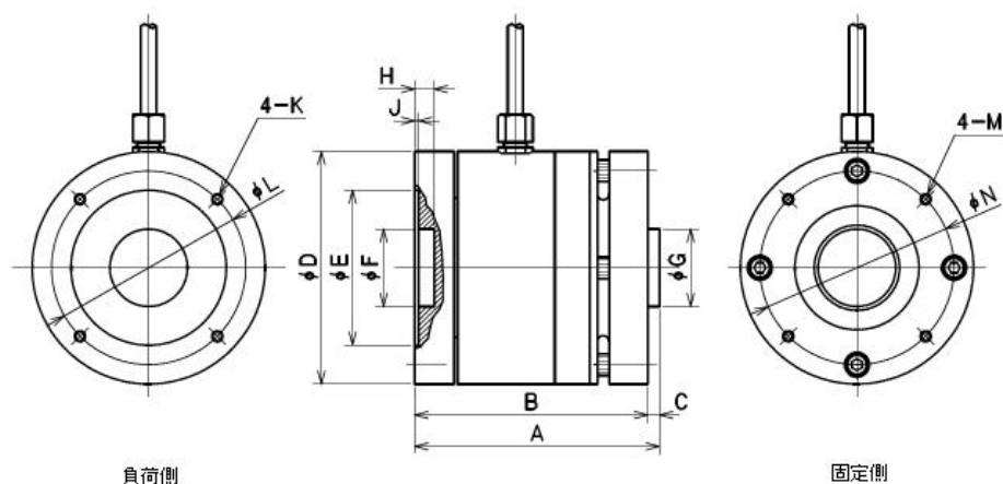
形式名と定格・寸法・質量(単位:mm)
