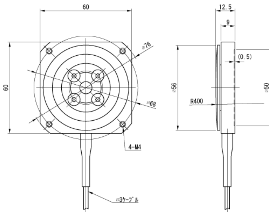
寸 法 图
