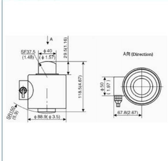
外型尺寸 mm(inch)
