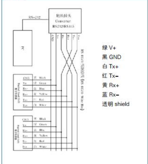
接线方式
