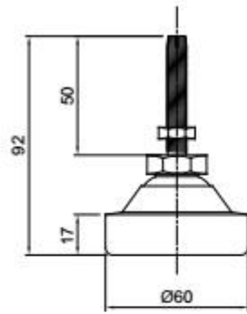
PIEDINOSB2M8 M8x1.25
