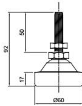
PIEDINOSB2INOX M12x1.75
