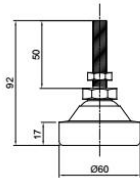
PIEDINOSB2M10 M10x1.5
