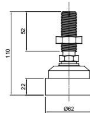
PIEDINOSB2ZNCM20 M20x2.5
