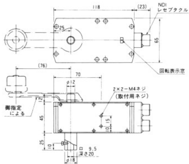
寸法図
