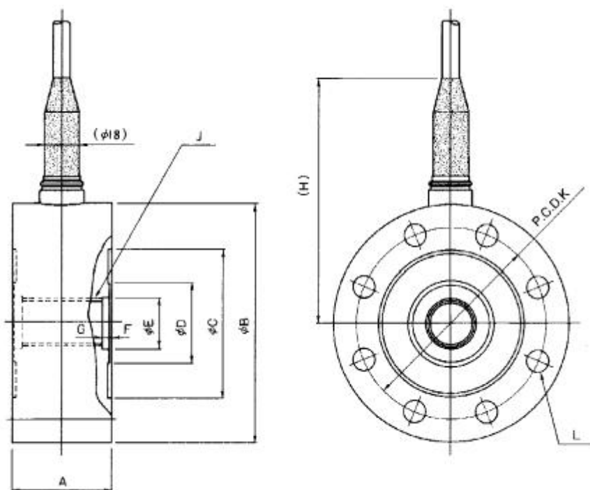
形式名と定格容量・寸法・質量(単位:mm)
