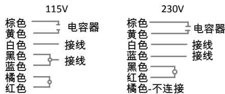
接线图
