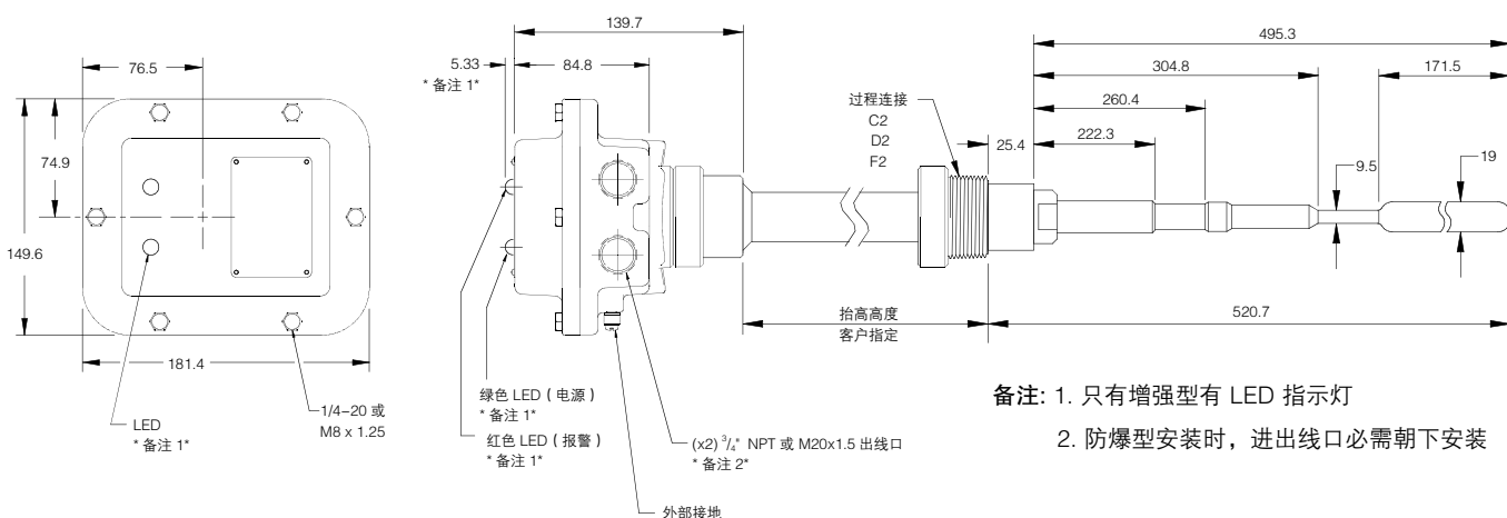
图示为飞灰探杆使用 C2、D2&F2 型过程连接
