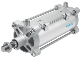
气缸 DSBG-160-300-PPVA-N3
