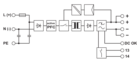
结构框图
