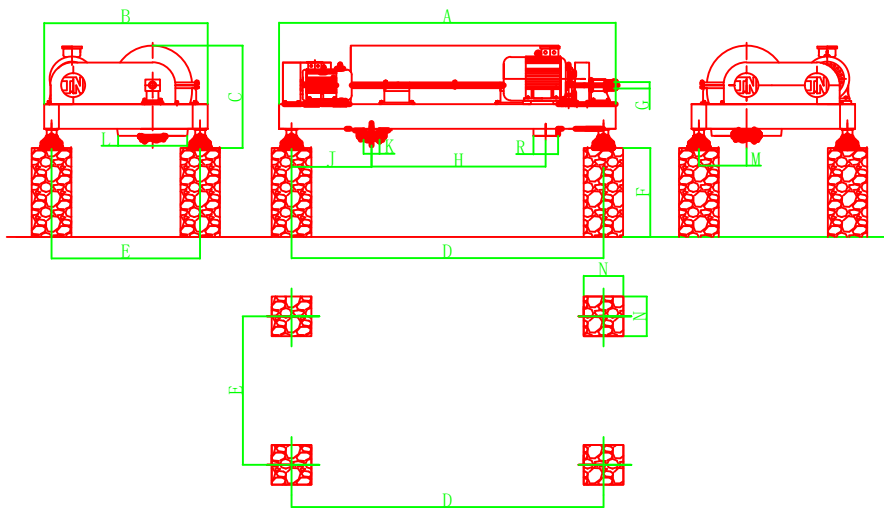
LWJ系列离心机外形尺寸及底座基础参数图
