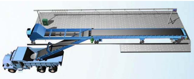
图 4. 可用于水泥厂高台装车机
